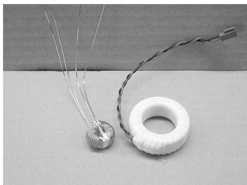
磁気増幅器M-TYPE
